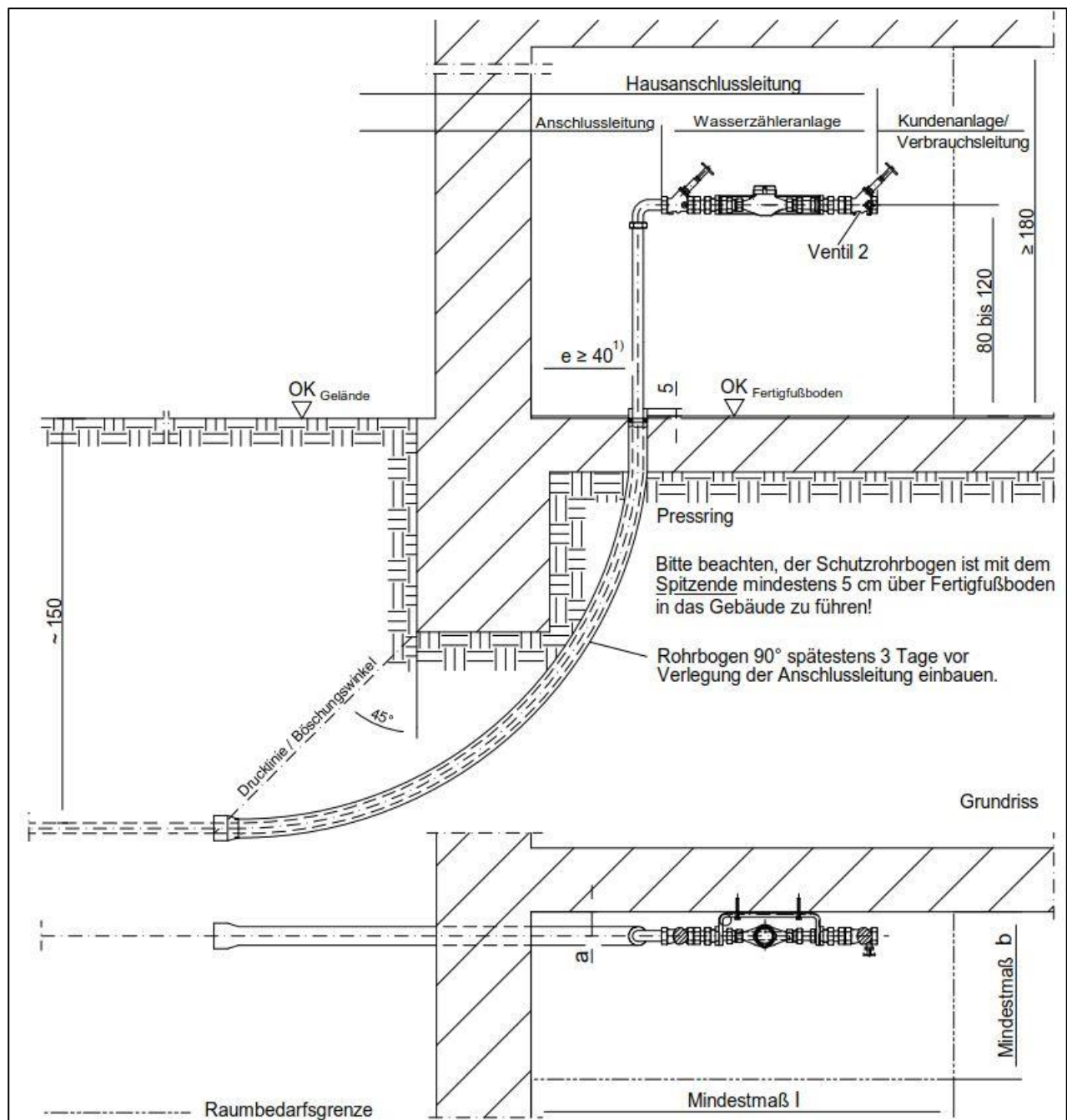
Bild 2 – Einbauraum für die Wasserzähleranlage im Hauswirtschaftsraum im Gebäude ohne Keller für Anschlussleitung aus PE (Prinzipische Skizze)
